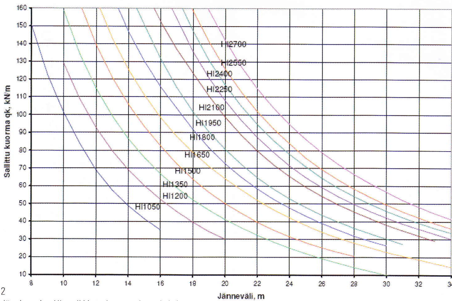
HI-palkkien kantavuuskäyrät B = 480mm
